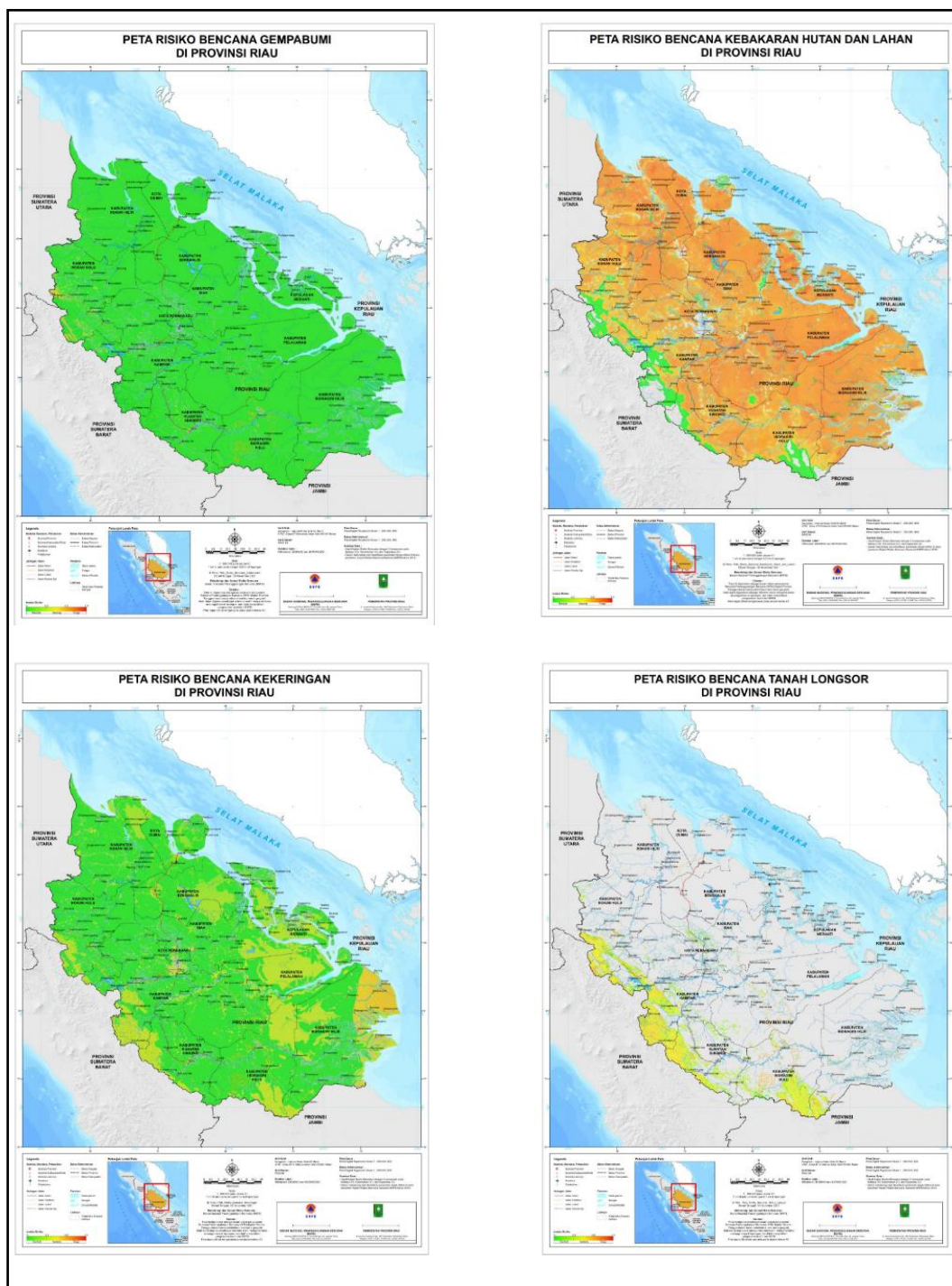
Gambar 2.4 Peta Risiko Gempa Bumi, Karhutla, Kekeringan dan Tanah Longsor Di Provinsi Riau
