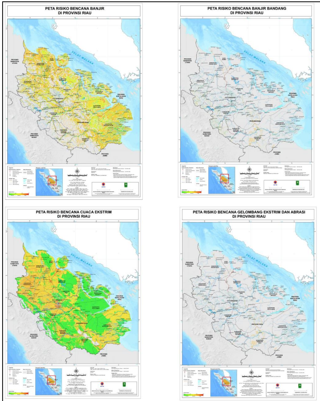
Gambar 2.3 Peta Risiko Bencana Banjir, Banjir Bandang, Cuaca Ekstrem dan Abrasi Di Provinsi Riau
